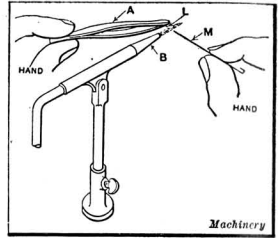
Fig. 15. Welding Tungsten and Platinum Wires
